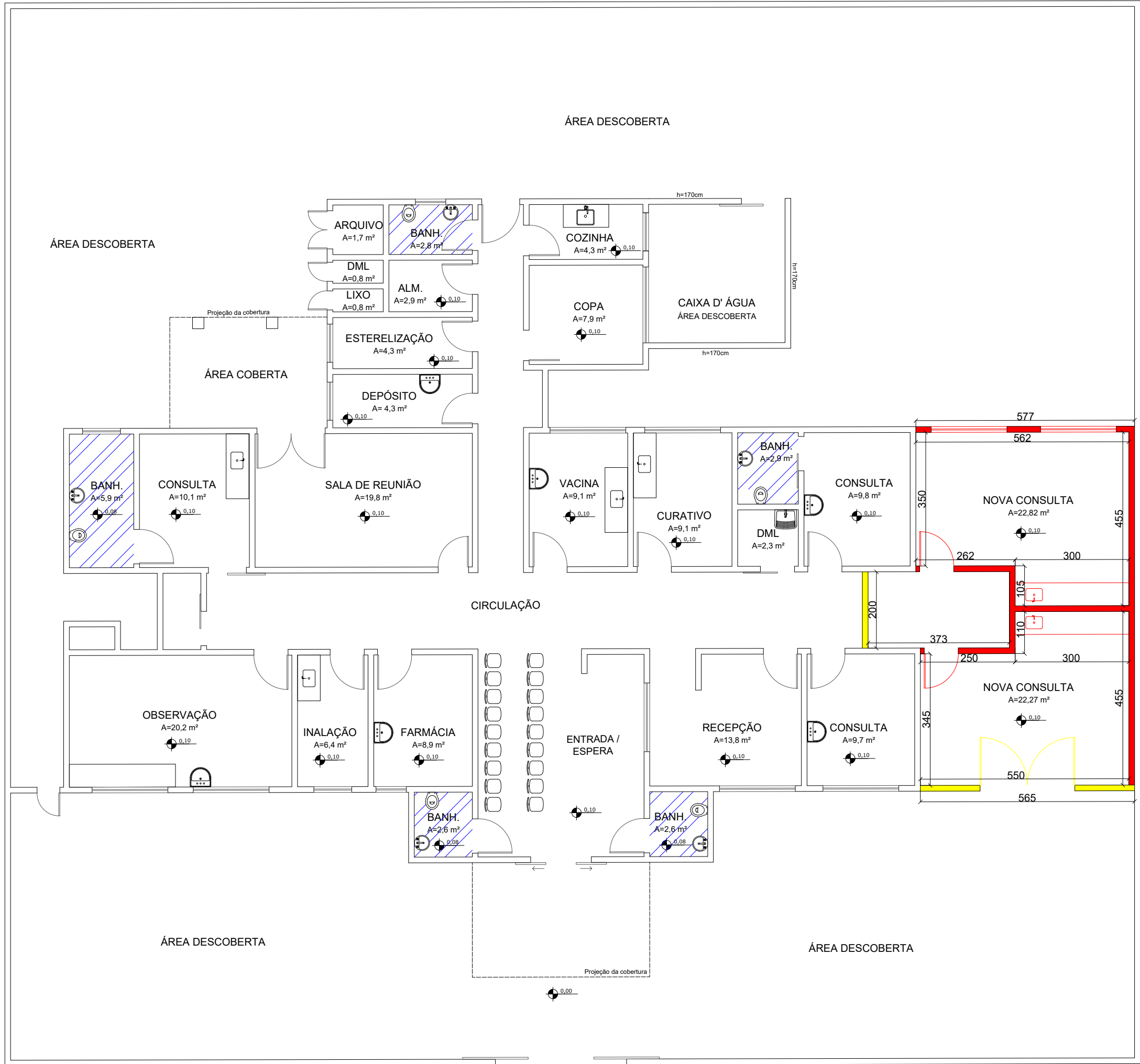
PLANTA BAIXA INICIAL ESCALA 1:100
